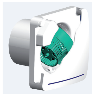
Wentylator promieniowy wirnik z łopatkami pochylonymi do przodu, bardzo niski poziom hałasu.
