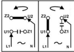
C B - Betriebskondensator
