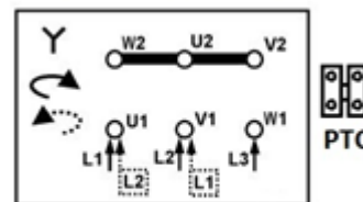
3x400V
