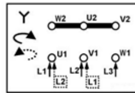
3x400V
