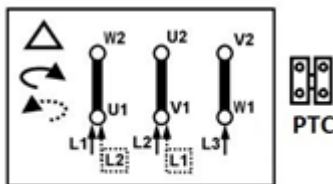
3x230V
