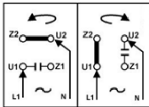
Dreieckschaltung
