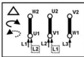
3x230V
